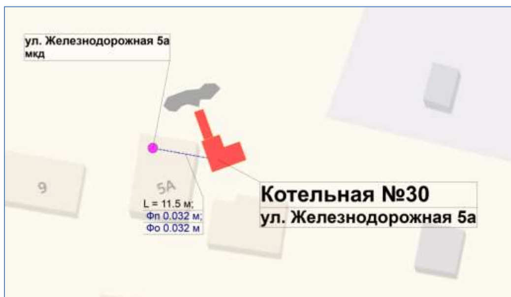
Рисунок 14. Схема тепловых сетей котельной № 30
