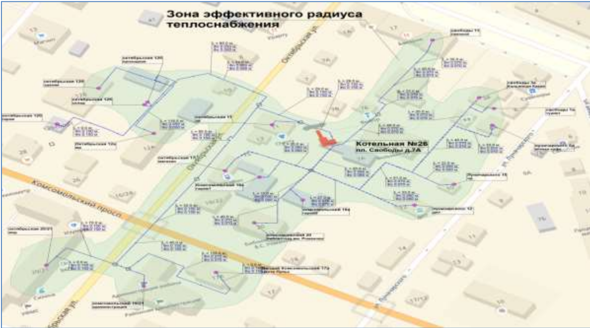
Рисунок 25. Зона эффективного радиуса теплоснабжения котельной № 26
