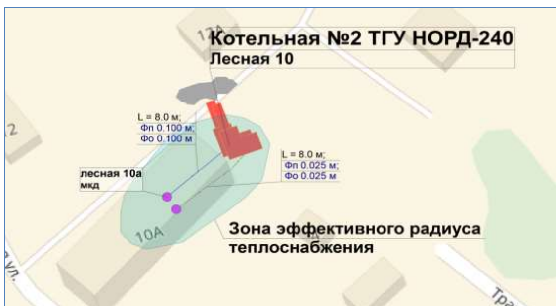
Рисунок 17. Зона эффективного радиуса теплоснабжения ТГУ Норд -240
