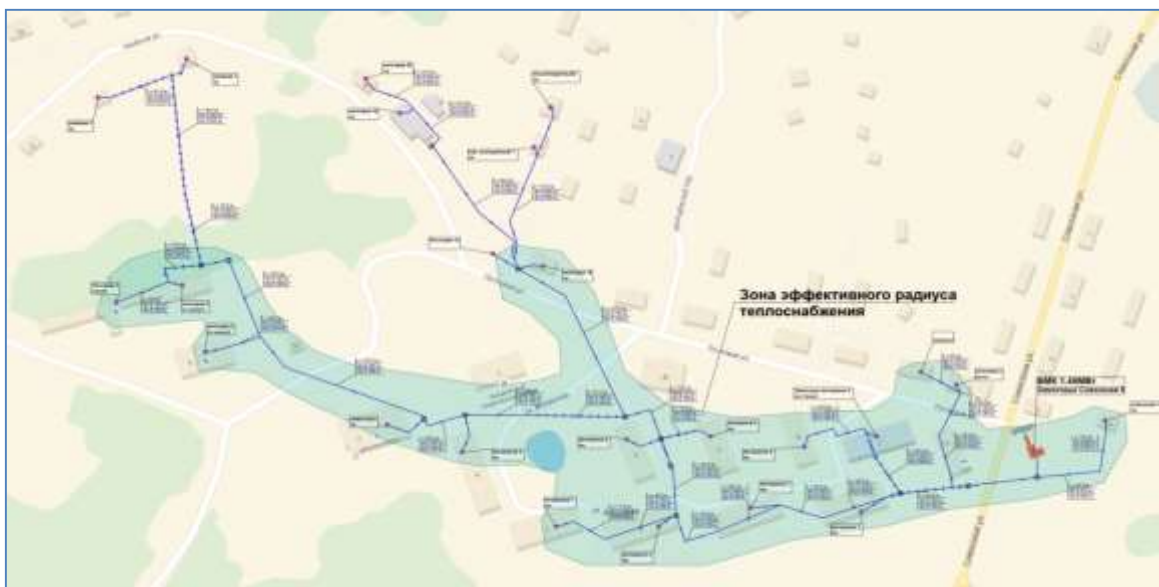
Рисунок 20. Зона эффективного радиуса теплоснабжения БМК 1.46 МВт
