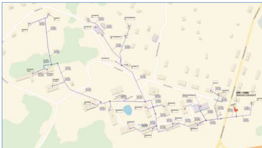
Рисунок 5. Схема тепловых сетей БМК 1,46 МВт
