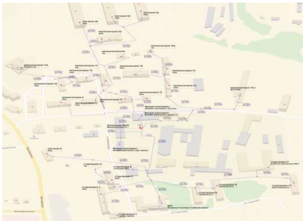
Рисунок 10. Схема тепловых сетей котельной № 12 г. Валдай ул. Механизаторов, д. 21
