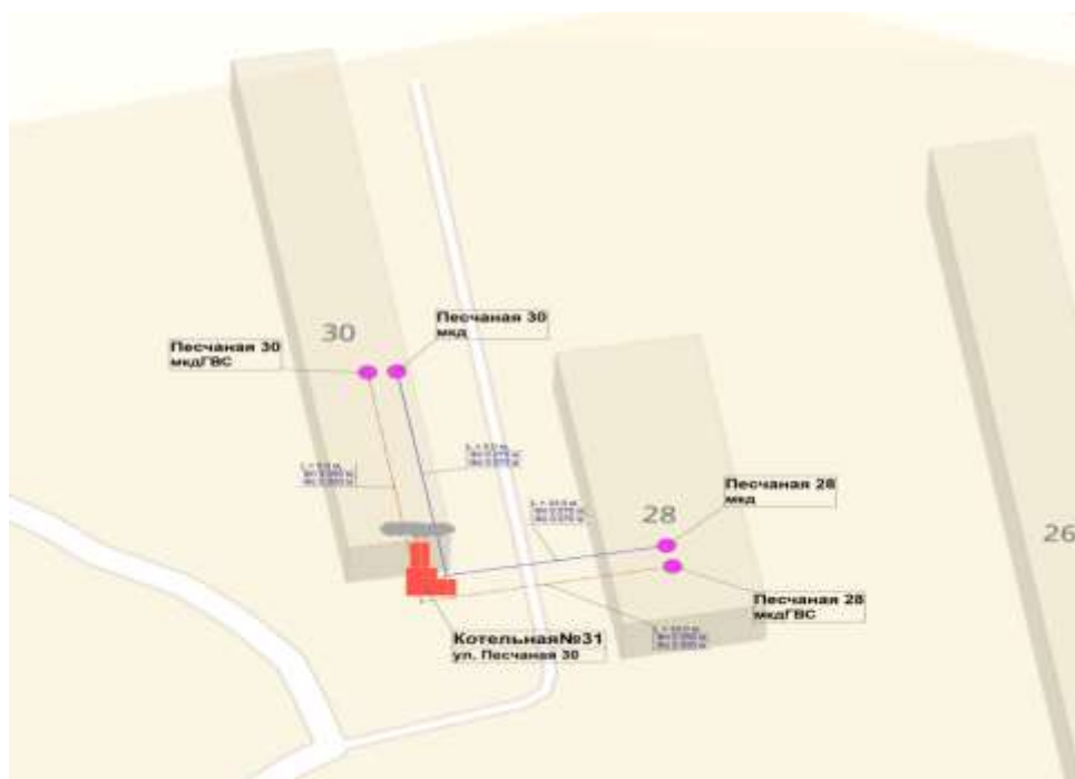
Рисунок 15. Схема тепловых сетей котельной № 31 г. Валдай, ул. Песчаная, д. 30
