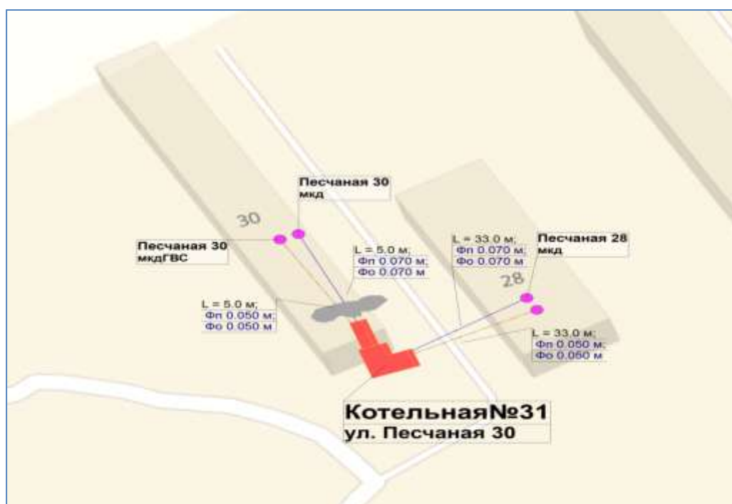
Рисунок 15. Схема тепловых сетей котельной № 31
