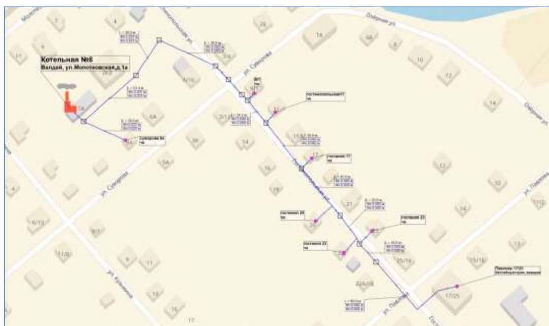
Рисунок 6. Схема тепловых сетей котельной № 8 г. Валдай, ул. Молотковская, д. 11а
