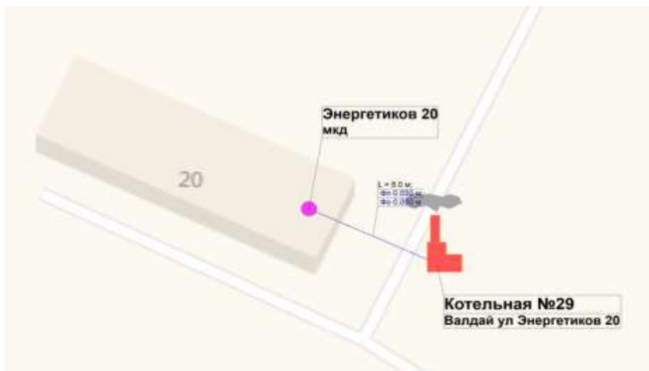
Рисунок 13. Схема тепловых сетей котельной № 29 г. Валдай, ул. Энергетиков, д. 20
