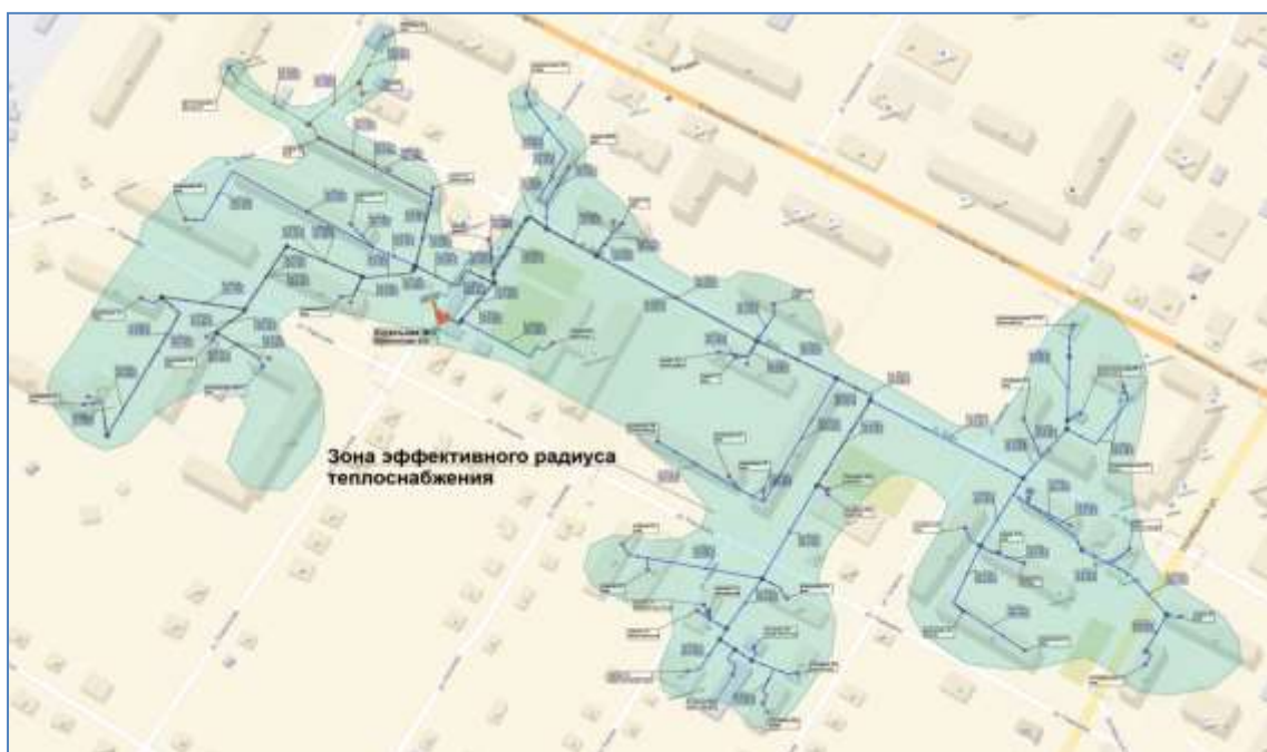
Рисунок 18. Зона эффективного радиуса теплоснабжения котельной № 3
