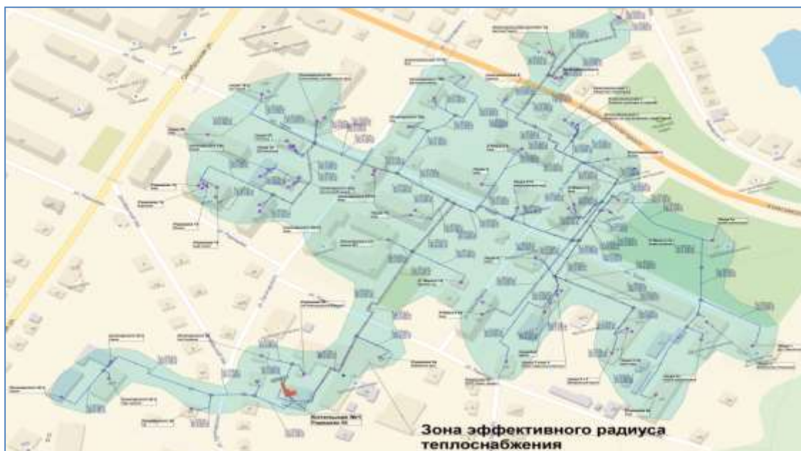
Рисунок 16. Зона эффективного радиуса теплоснабжения котельной № 1
