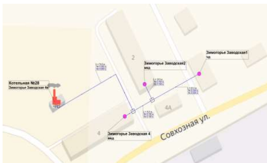
Рисунок 12. Схема тепловых сетей котельной № 28 Валдайский р-н, с. Зимогорье, ул. Заводская, д. 46
