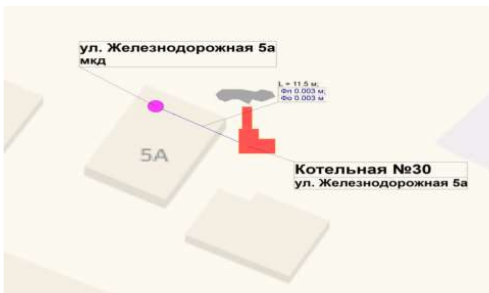
Рисунок 14. Схема тепловых сетей котельной № 30 г. Валдай, ул. Железнодорожная, д. 5а
