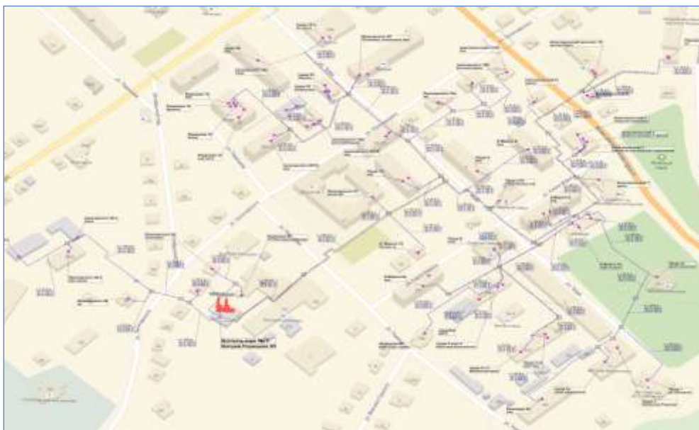
1. Схема тепловых сетей котельной № 1 г. Валдай ул. Радищева, д. 5б
