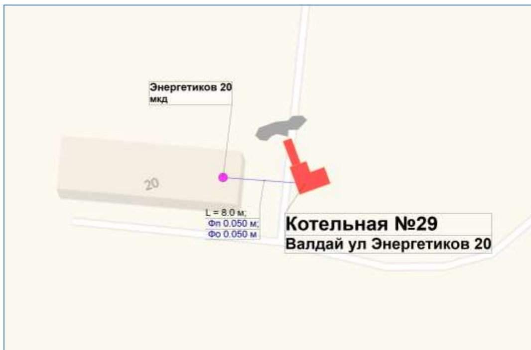
Рисунок 13. Схема тепловых сетей котельной № 29
