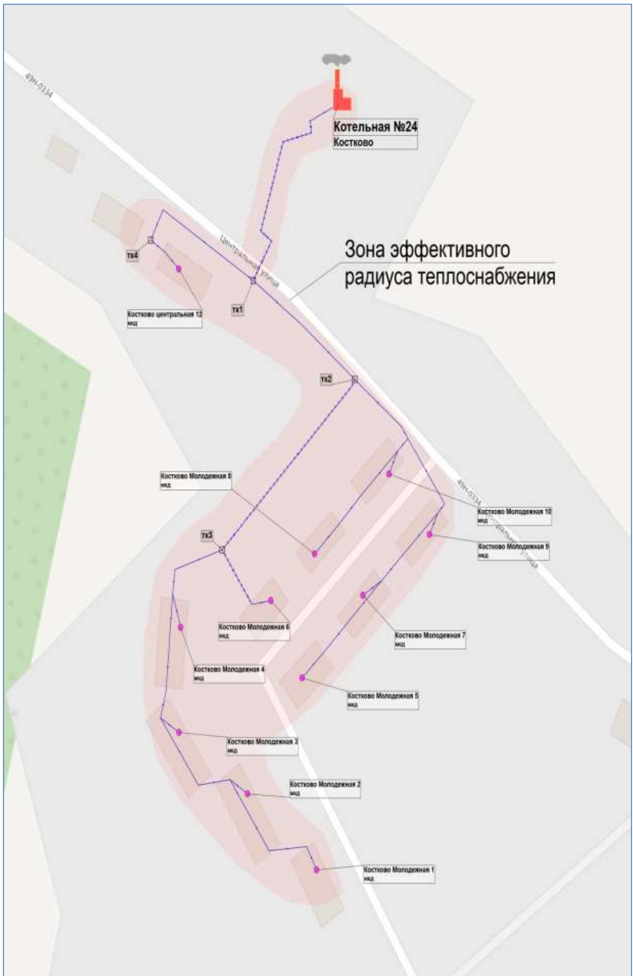
Рисунок 2. Зона эффективного радиуса теплоснабжения котельной № 24
