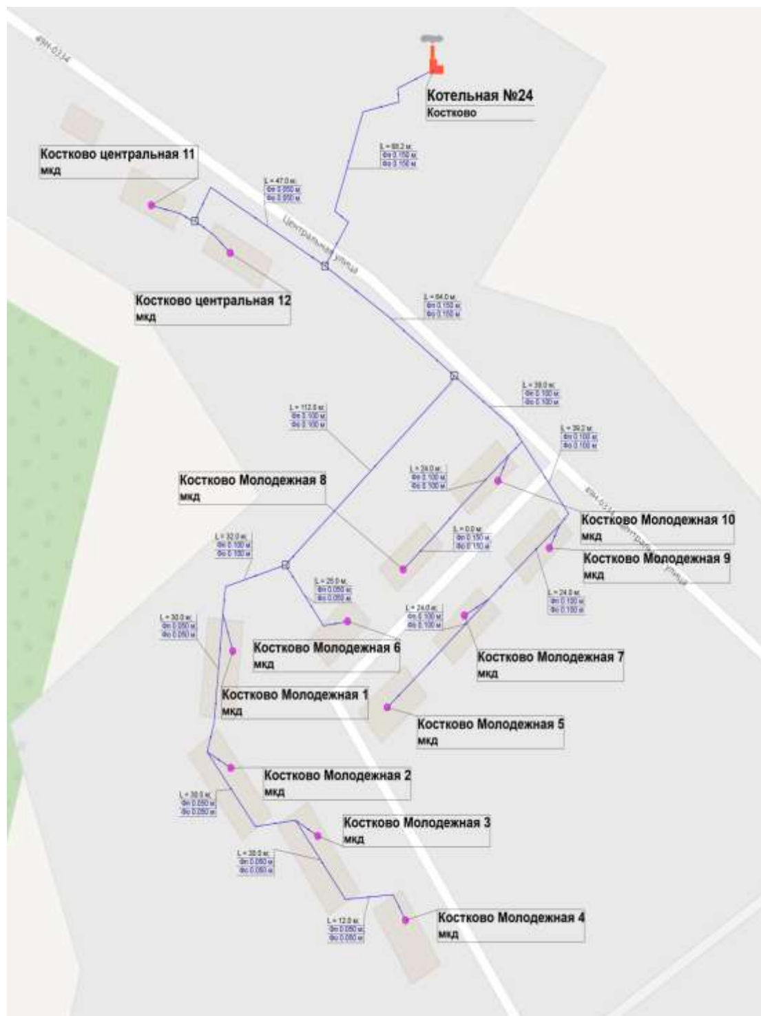
Рисунок 1. Схема тепловых сетей котельной № 24 д. Костково
