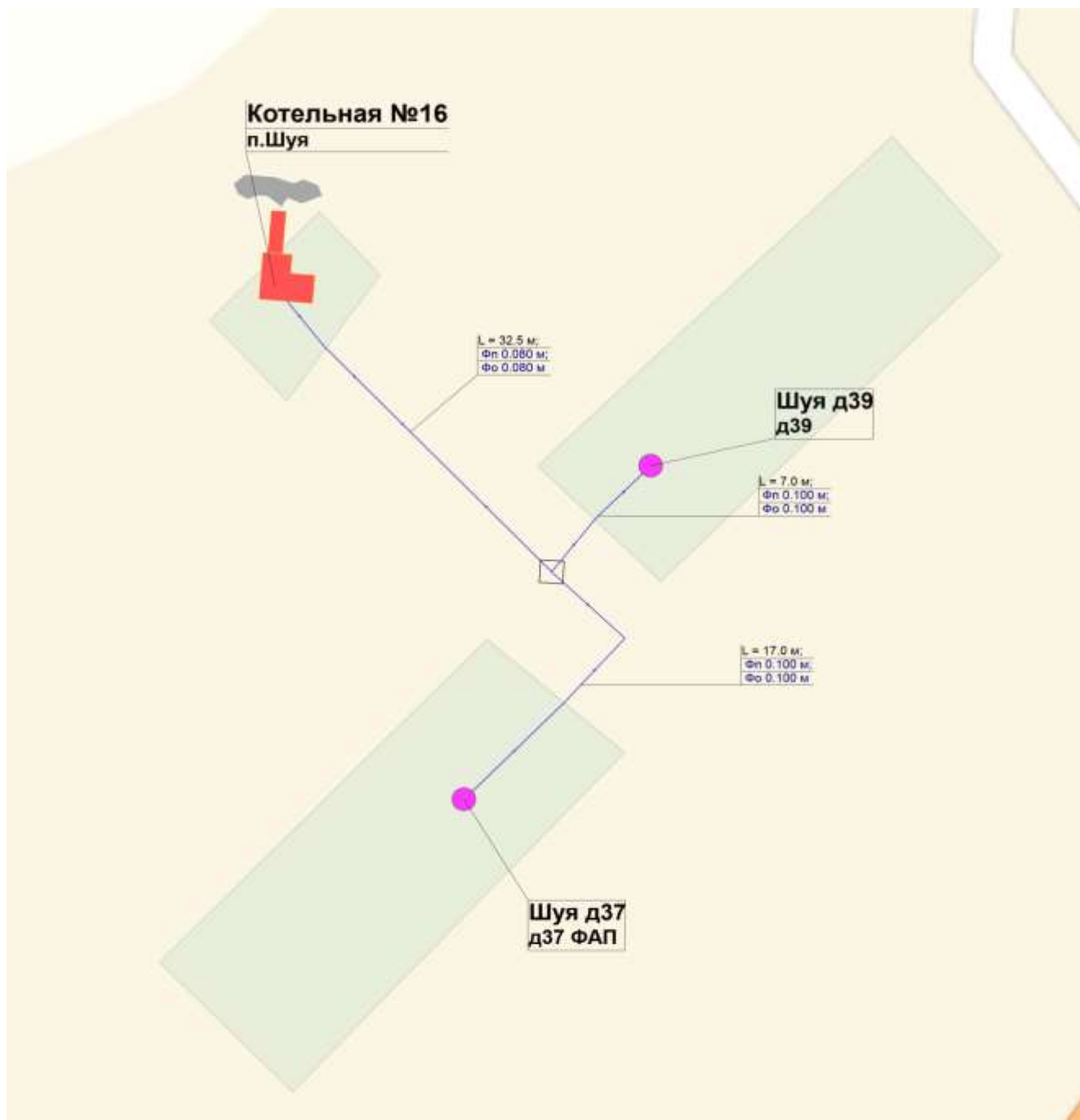
Рисунок 2. Схема тепловых сетей котельной №16 д. Шуя
