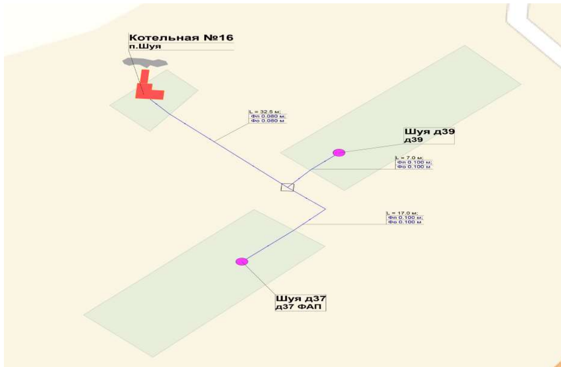
Рисунок 2. Схема тепловых сетей котельной № 16, д. Шуя
