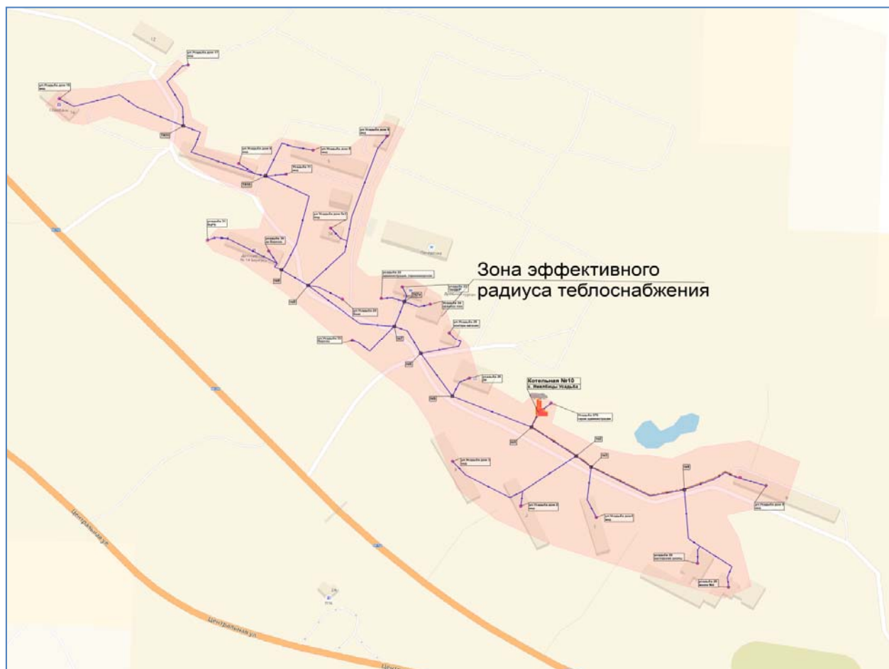
Рисунок 3. Зона эффективного радиуса теплоснабжения котельной №10
