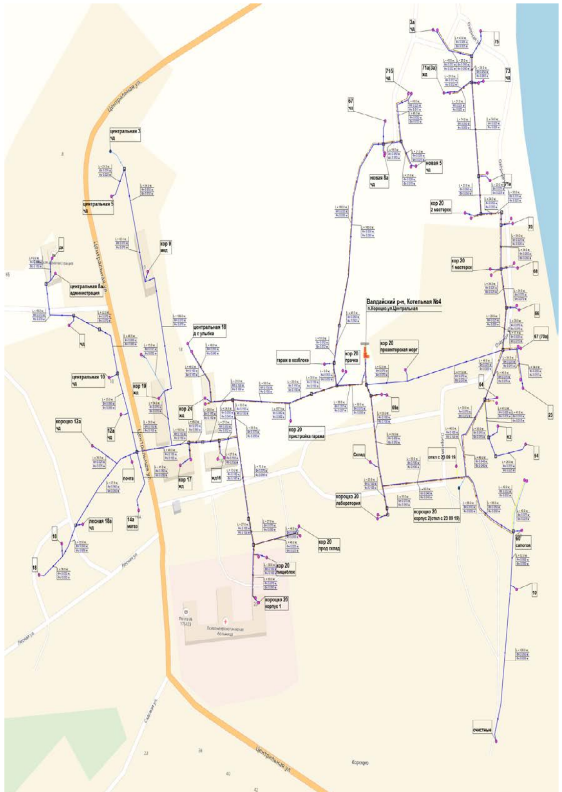
Рисунок 1. Схема тепловых сетей котельной № 4 п. Коротко, ул. Центральная
